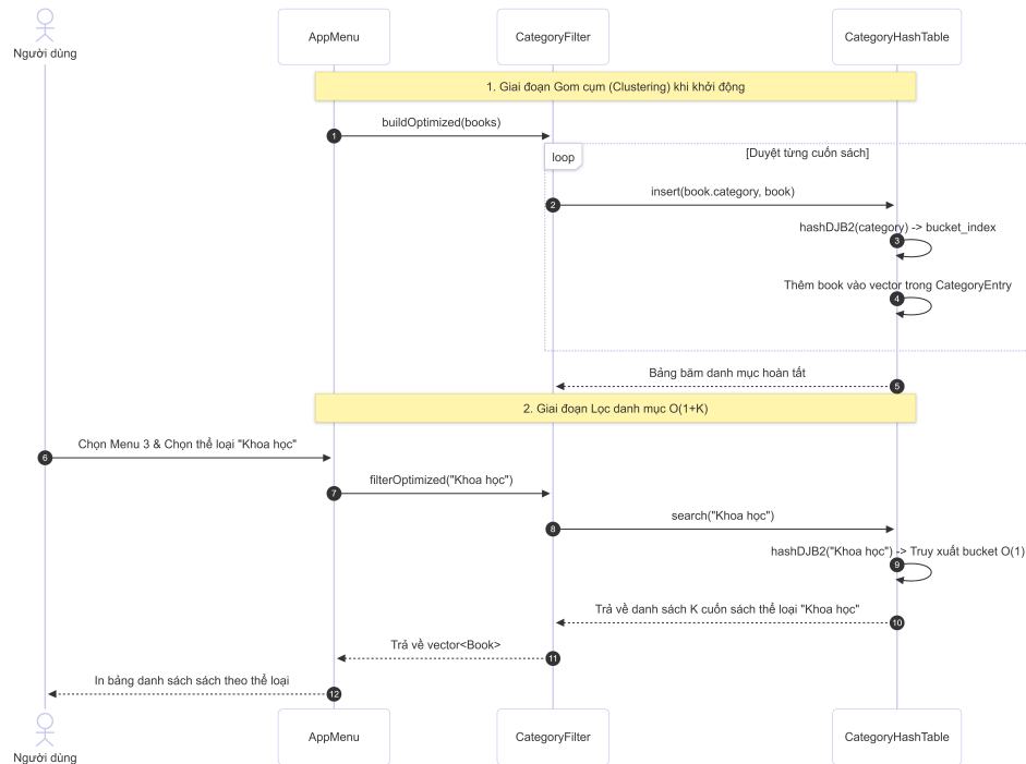
Hình 7. Sơ đồ tuần tự thể hiện luồng lọc sách theo thể loại (RQ1)
