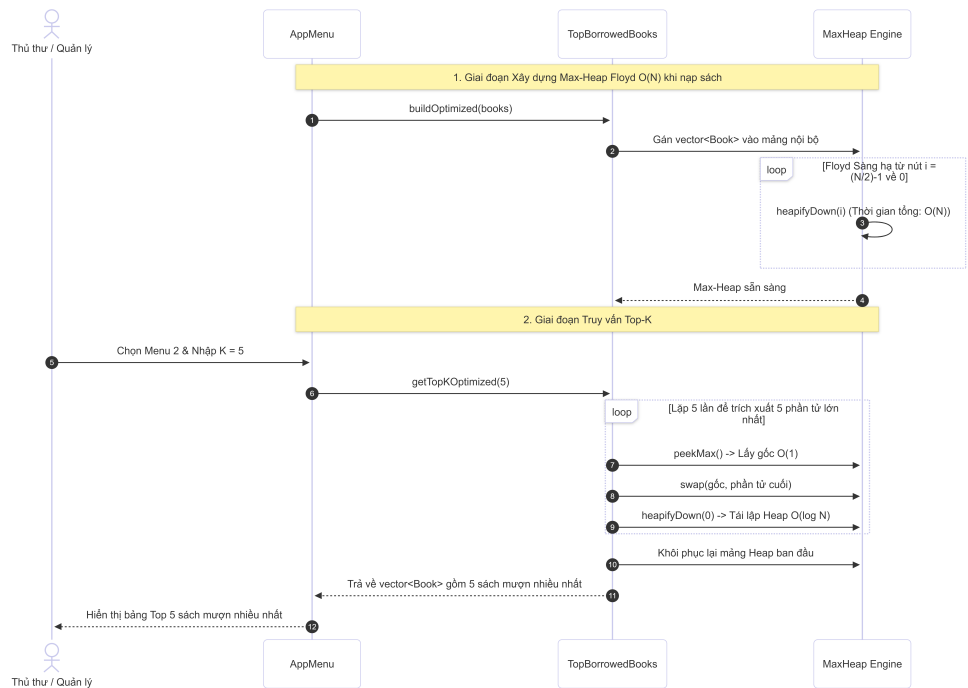
Hình 5. Sơ đồ tuần tự thể hiện luồng trích xuất sách mượn nhiều nhất (MC2)
