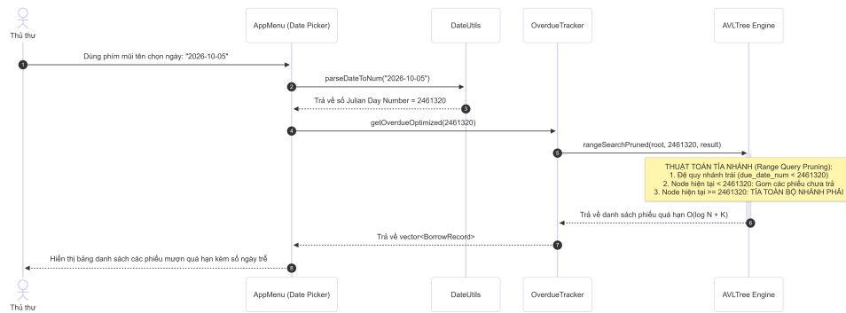
Hình 9. Sơ đồ tuần tự thể hiện luồng truy vết phiếu mượn quá hạn (RQ2)
