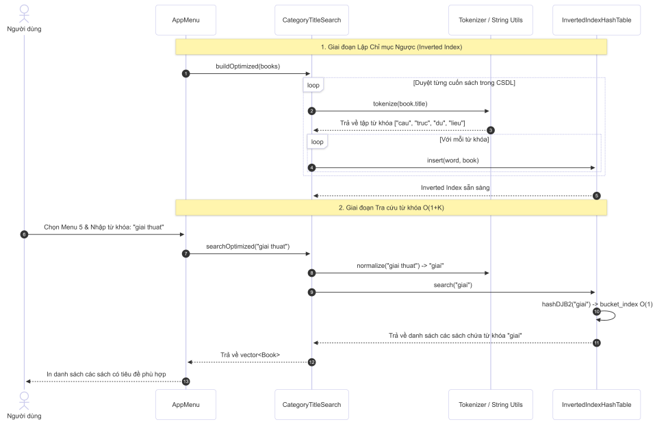
Hình 11. Sơ đồ tuần tự thể hiện luồng tìm kiếm tựa sách theo từ khóa (RQ3)
